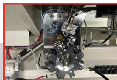
CAMBIO SPOLA AUTOMATICO AUTOMATIC BOBBIN CHANGER
